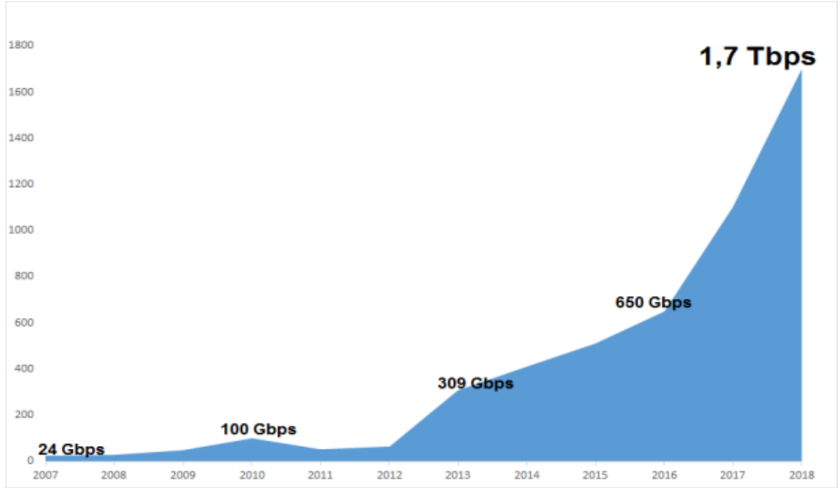
Şekil 1. Raporlanan en yüksek DDoS saldırı boyutları( Arbour Networks, 2017)
